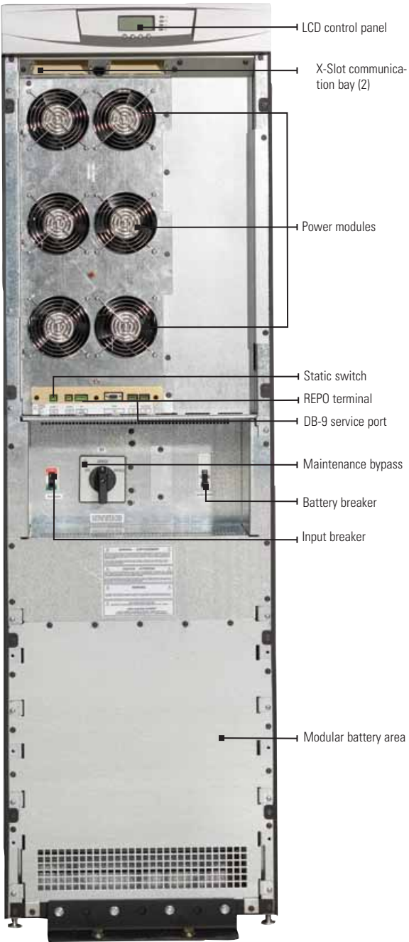
20/30 kVA UPS
